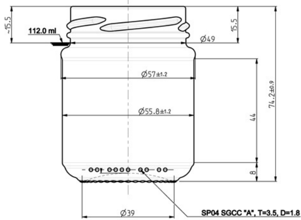
Back view (Widok z tyłu)
