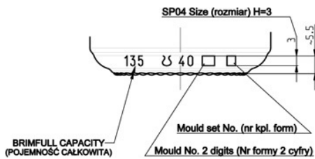
Front view (Widok z przodu) Developed view of description (Opisy w rozwinięciu)
